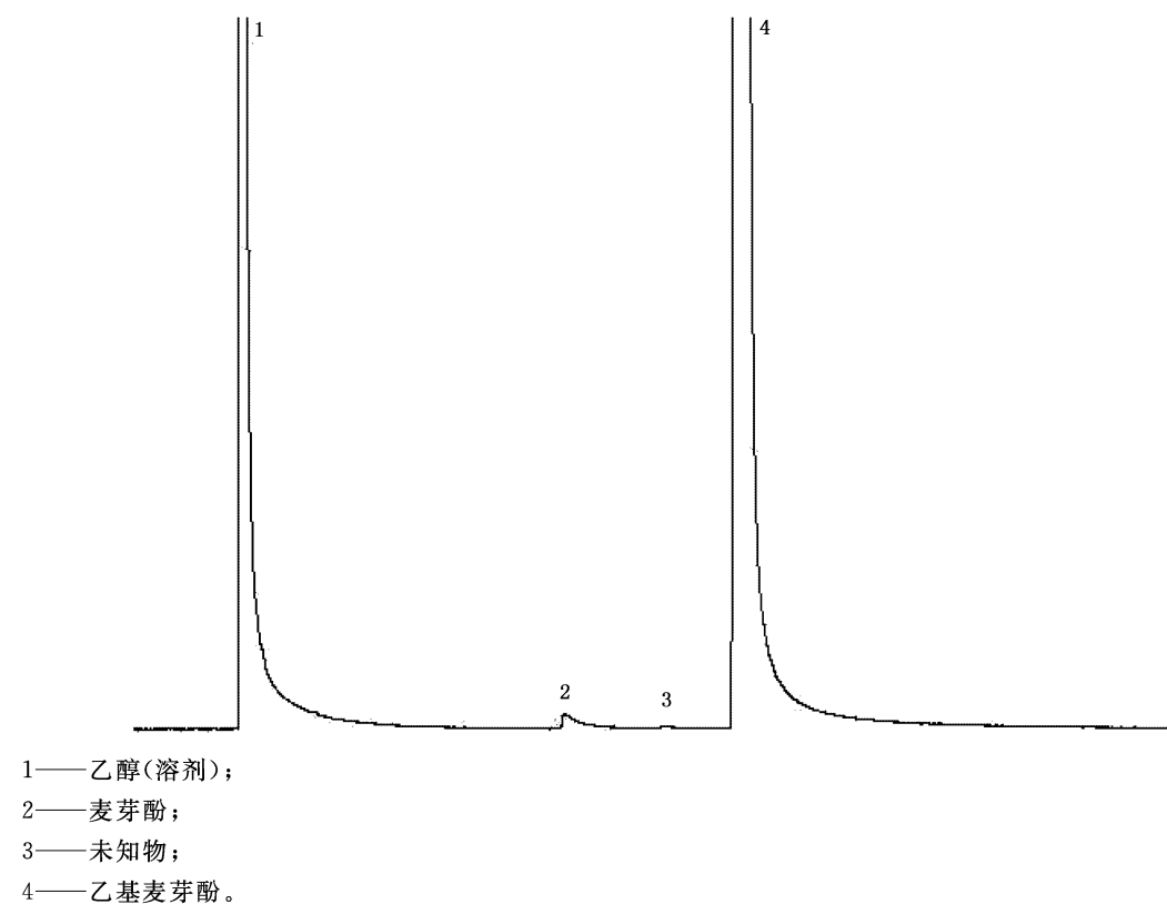
图 B.1 乙基麦芽酚含量毛细管柱典型色谱图
